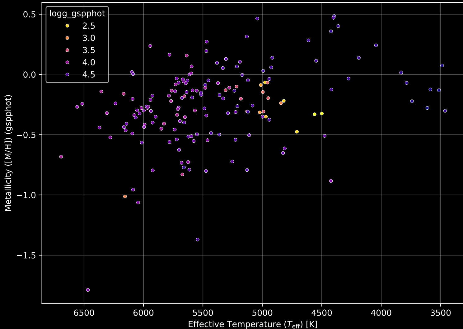
APOGEE DR17 Field: [JHelum5] Stellar Population Parameters (n= 165)
